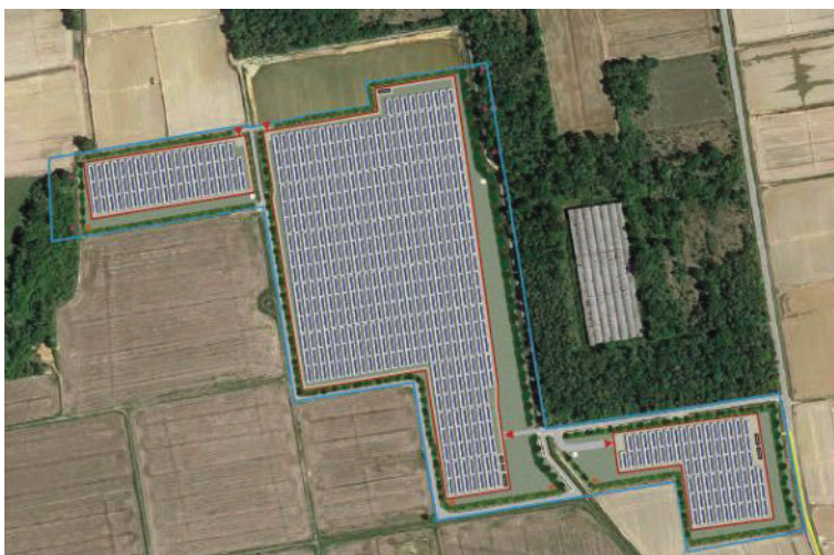
Figura 2: Layout del campo fotovoltaico e dettaglio delle opere di mitigazione, estratto da R_7.1_ROA_OMA_0-Opere di mitigazione e compensazione ambientale_R1 Rev. 2 – luglio 2025
